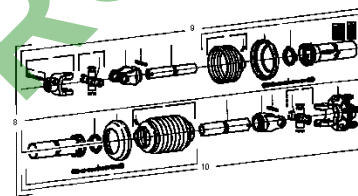
ETB-008699, Wałek przekąźnikowy
