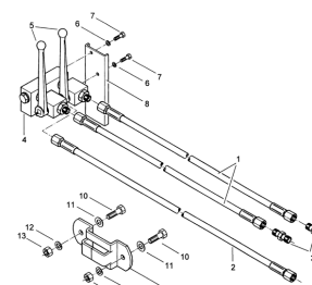
ETB-008691, Zespół dwudrogowy
