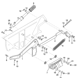
ETB-008685, Dźwignia nastawcza i zsypy z lewej strony
