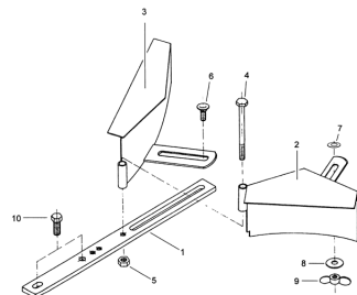
ETB-008694, Urządzenie do rozsiewu rzędowego do upraw owoców
