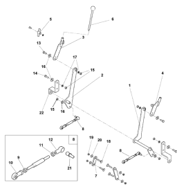
ETB-008700, Sterowanie ręczne
