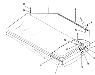
ETB-008692, Składana plandeka
