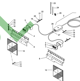
ETB-008696, Oświetlenie tylne
