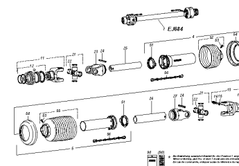
ETB-0000005672, Wałek przegubowo-teleskopowy EJ684 -W 100 E 710 mm, 1 3/8 cala, 6 sztuk
