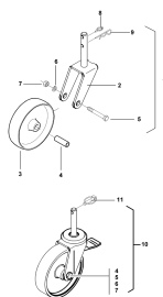
ETB-008697, Urządzenie transportowe i postojowe
