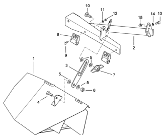
ETB-008693, Ekran rozsiewu granicznego
