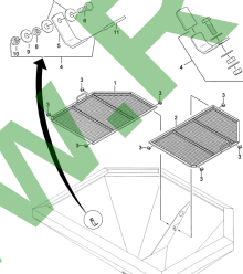
ETB-008690, Sito chroniące przed ciałami obcymi, składane
