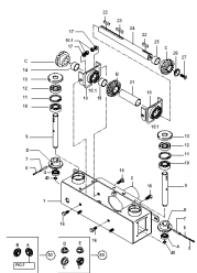
ETB-008689, Przekładnia (2/2)
