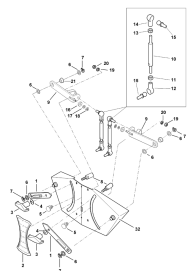
ETB-008686, Skala ilości
