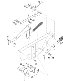
ETB-008684, Dźwignia nastawcza i zsypy z prawej strony
