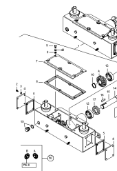
ETB-008688, Przekładnia (1/2)
