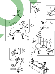
ETB-008687, Tarcze rozsiewające
